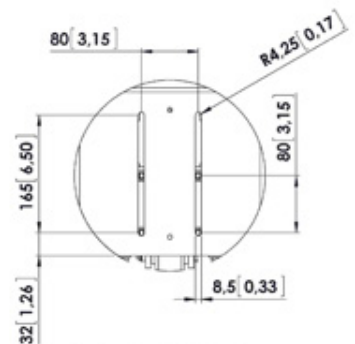
DETTAGLIO A SCALA 1 : 5
